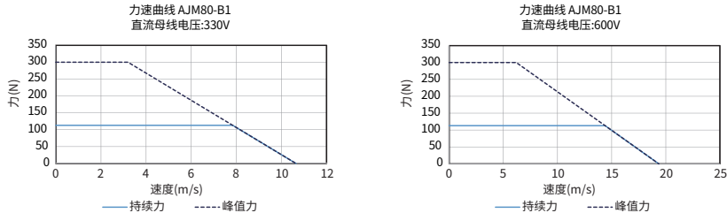
■ 力-转速 曲线
