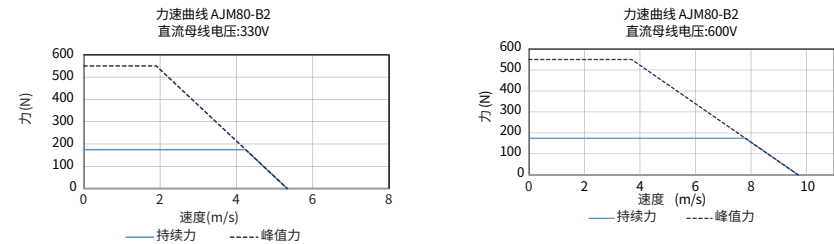
■ 力-转速 曲线
