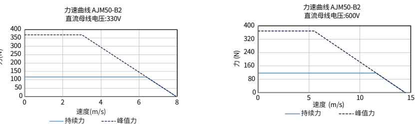
■ 力-转速 曲线
